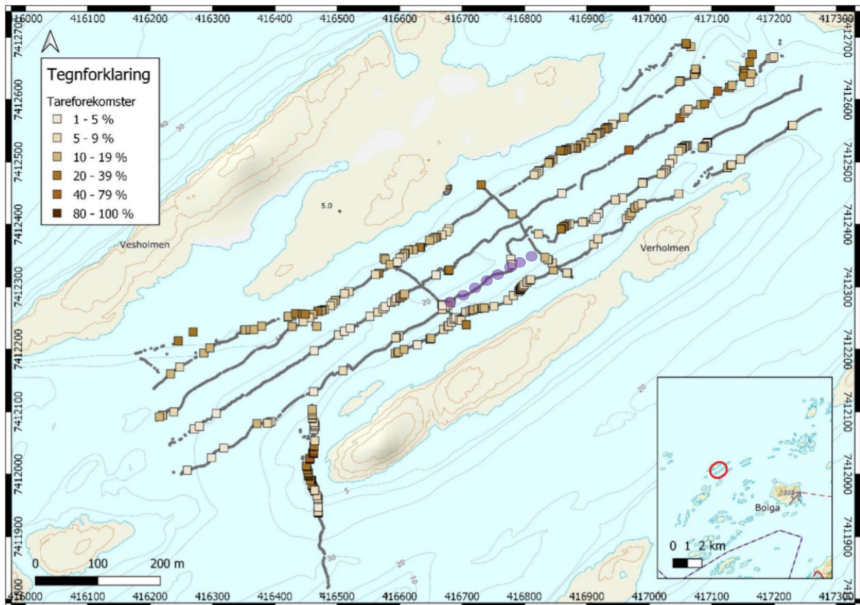
Figur 6. Prosentvis dekning av tareforekomster langs transektene ved Verholmen. Artsbestemmelse var utfordrende og derfor er alle artene (sukkertare, fingertare, stortare) poollet i figuren. De halv-gjennomsiktige punktene indikerer de 8 avløpsrørene. Figur fra Kartleggingsrapporten Verholmen 16 .
